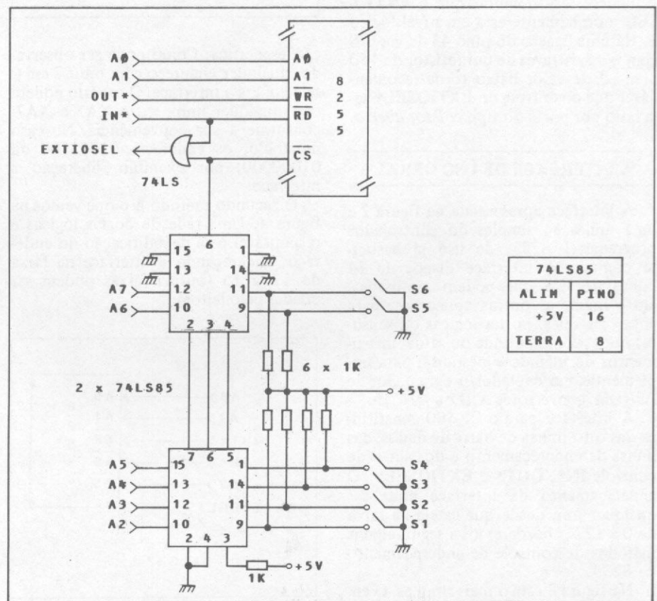
Figura 7 - Seleção por comparador programável
